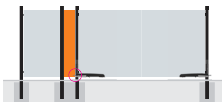
Darstellung eines Einzeltors mit einem elektrisch betriebenen Doppeltor und einem Element als Abstandhalter (benötigter Raum für den auf der Torinnenseite liegenden Elektro-Antrieb).
