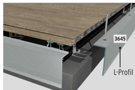
Beispiel mit seitlich und frontal angebrachten Rahmen L-Profilen.
